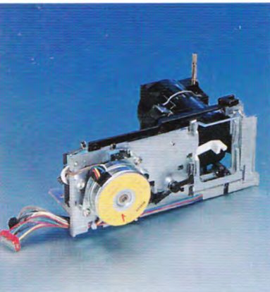
Modulo in pressofusione di zinco con vano caduta diapositive e portaobiettivo
