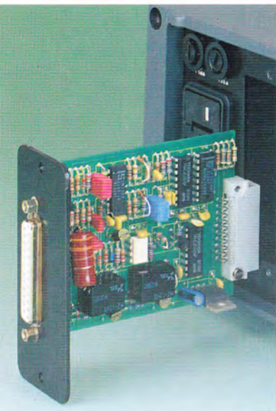
Modulo a 12/7 poli KODAK EKTAPRO (accessorio)
