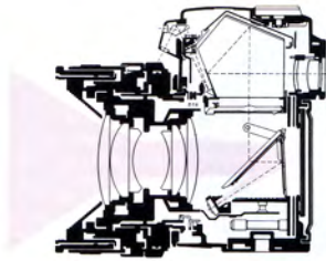
Rappresentazione schematica della misurazione integrale LEICA a tutto campo
